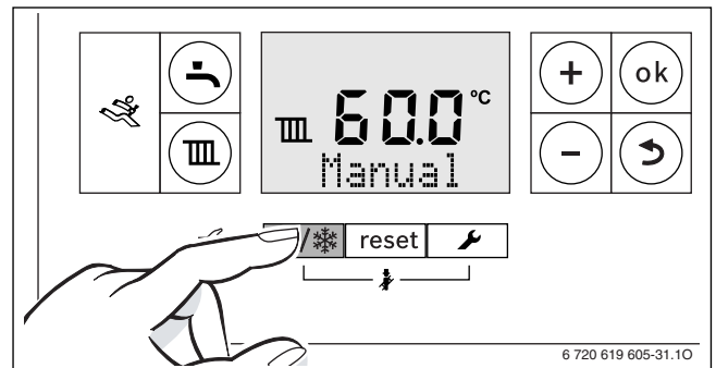
Fig. 41 Setarea regimului manual
