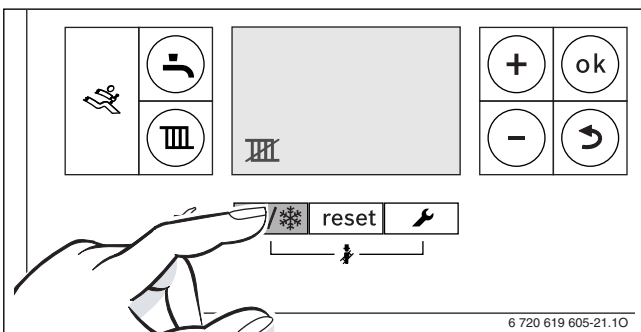
Fig. 39 Pornirea regimului de vară manual
